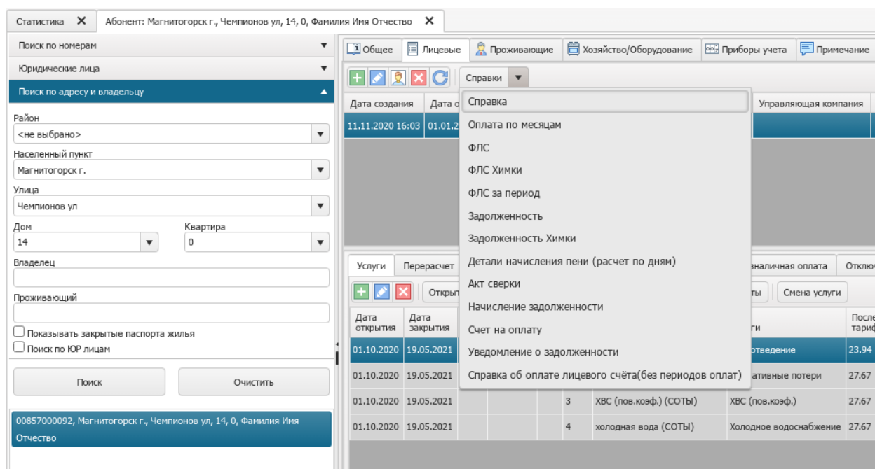
Рисунок 7.17 – Меню справки
