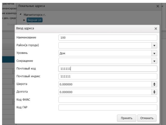
Рисунок 6.2 – Добавление дома
