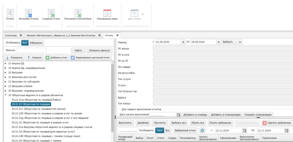
Рисунок 8.5 – Раздел «Отчеты»
