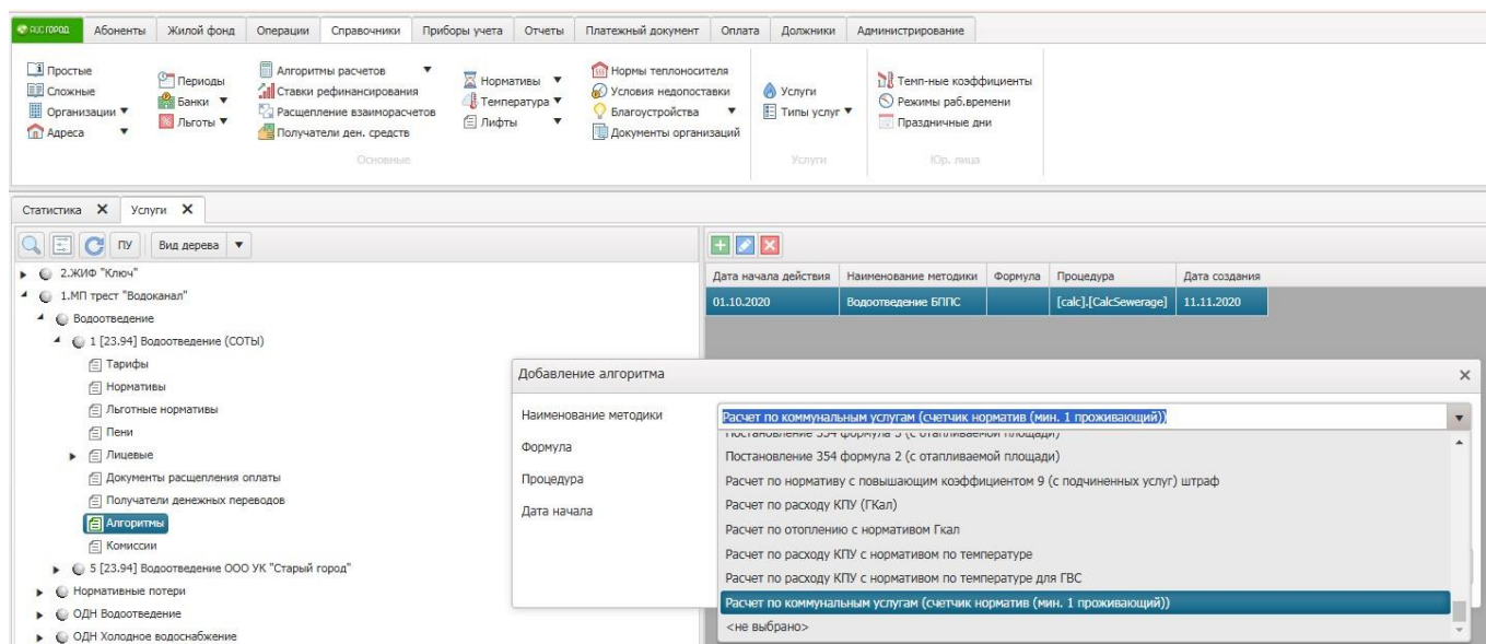
Рисунок 5.6 – Добавление алгоритма
